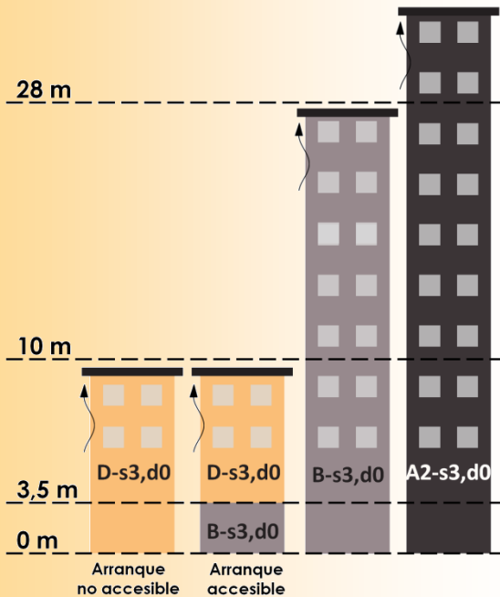
Exigencias del CTE para los sistemas de aislamiento de fachada ventilada.
