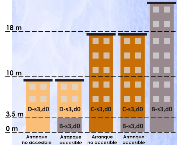
Exigencias del CTE para los sistemas constructivos de fachada.
