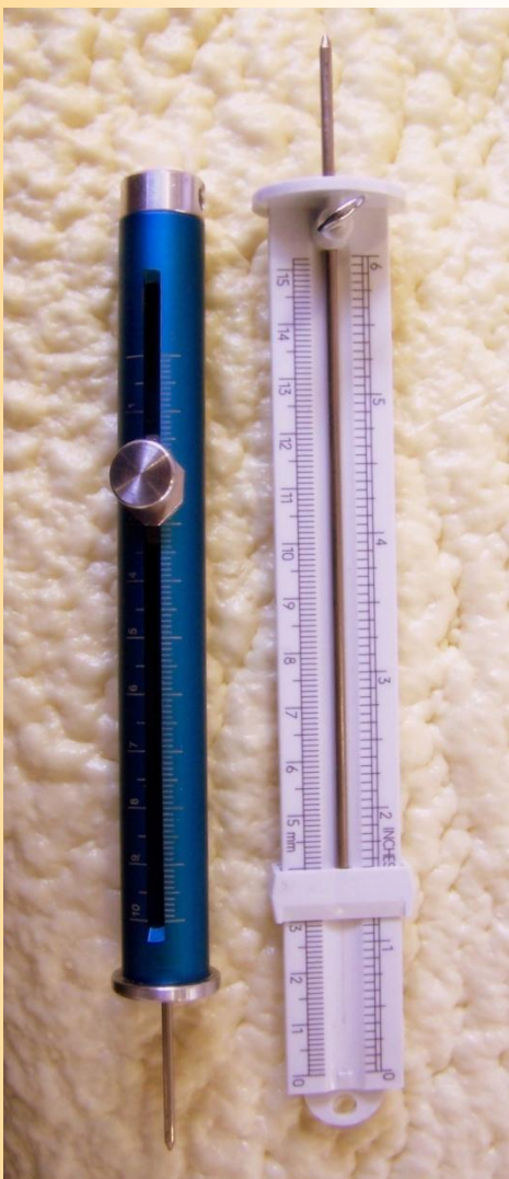
Punzones para medir el espesor del poliuretano proyectado.
