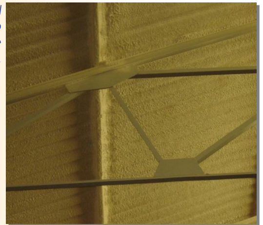
Proyección por el interior, envolviendo la estructura de soporte.
