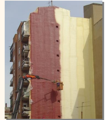
Proyección en medianera con protección
