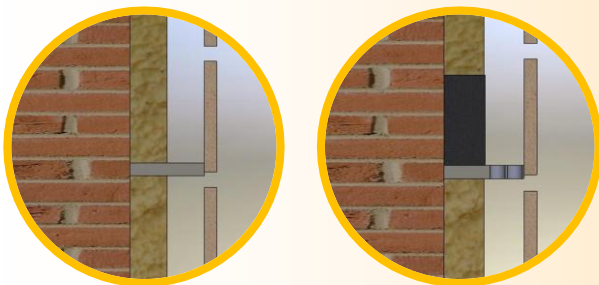
Compartimentación con barreras cortafuego intumescentes y no intumescentes. Ver capítulo 2.5
