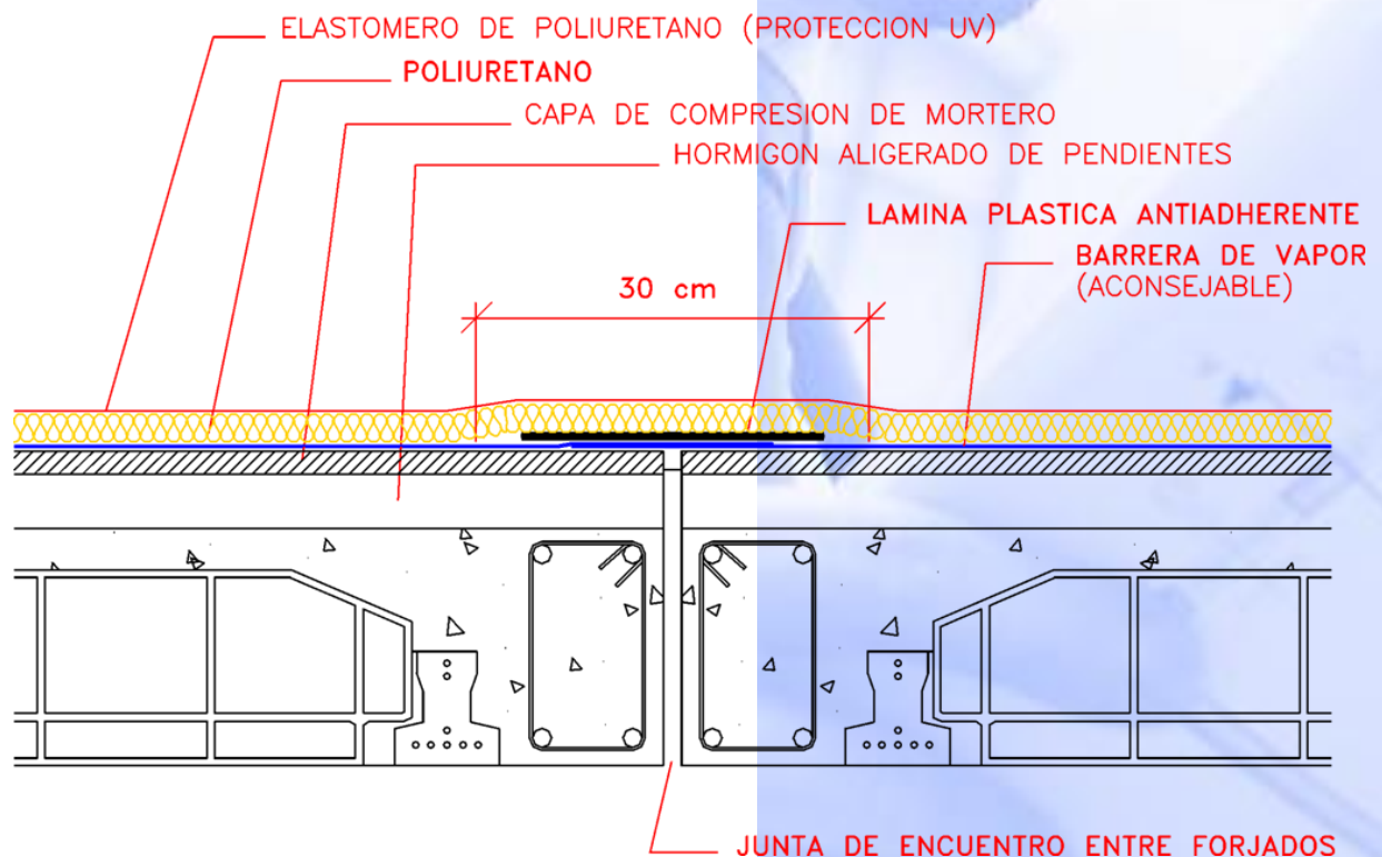
Tratamiento de una junta de dilatación en una cubierta plana con una banda elástica de al menos 30 cm de anchura.
