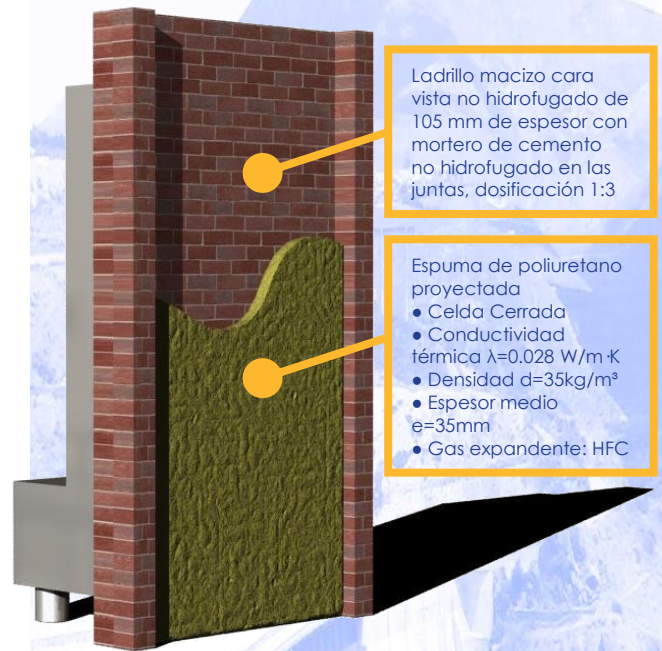
Solución constructiva ensayada para cumplir con la máxima exigencia de impermeabilidad.
